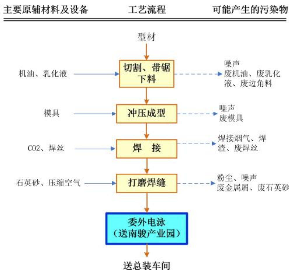
图4.3-13 电瓶架生产工艺及产污位置图
