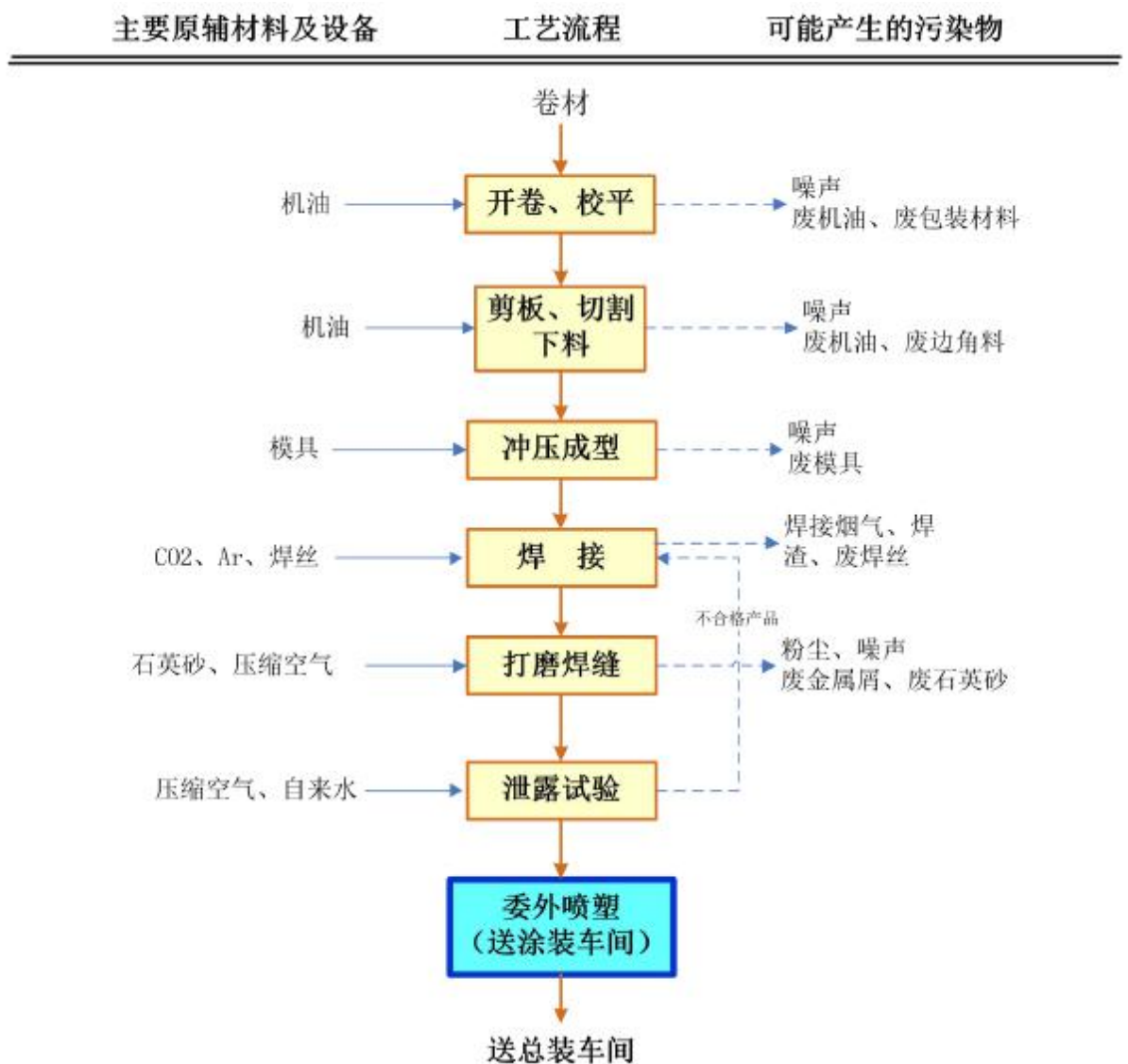
图4.3-12 储气罐生产工艺及产污位置图
