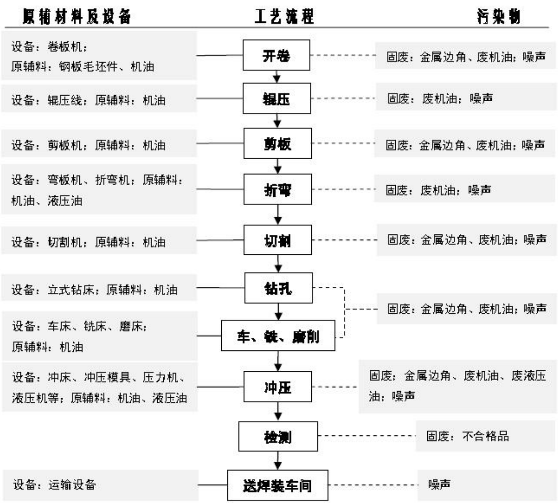
图4.3-3 成型车间工艺流程及产污位置图
