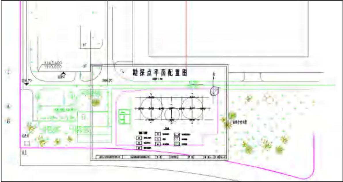
图 3.2-3 勘探点平面布置图
