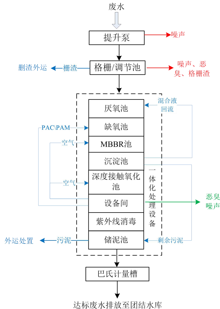
图 2-2 污水处理工艺流程及产污环节图
