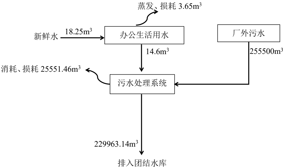
图 2-1 项目营运期水平衡图 m 3 /a
