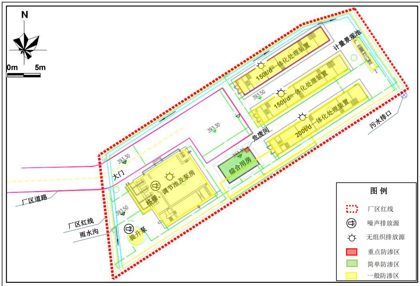
附图2-2 项目平面布置图
