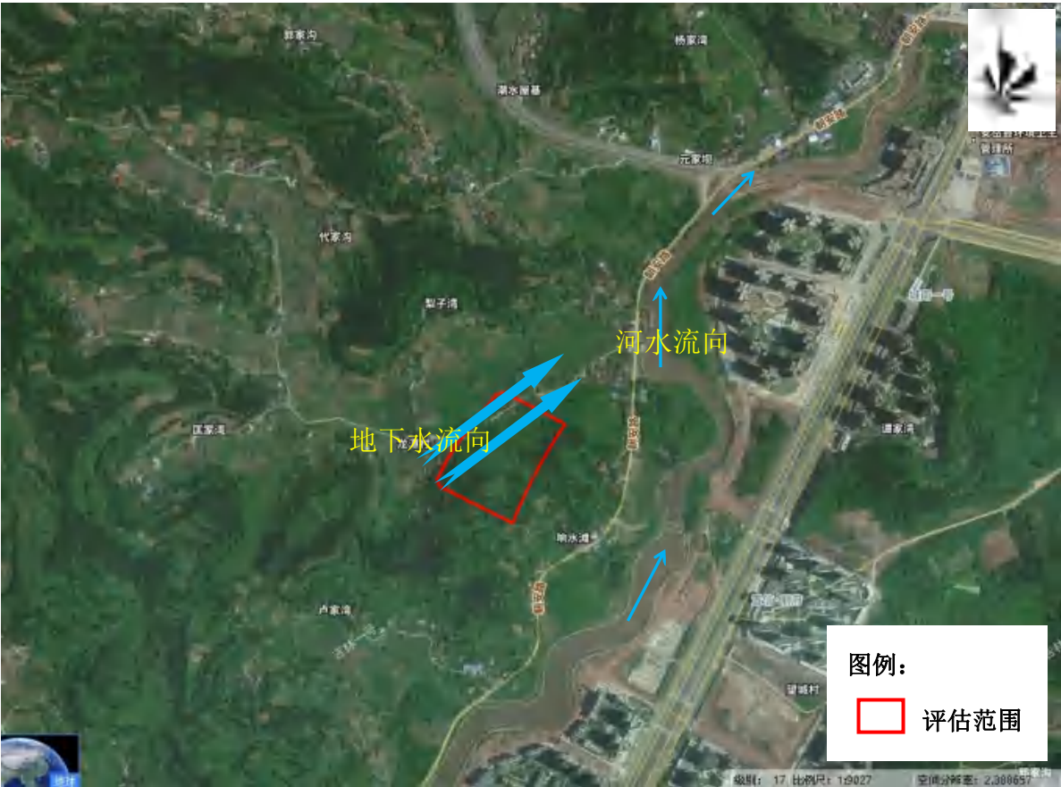
图 4.2-3 评价地块地下水流向图
