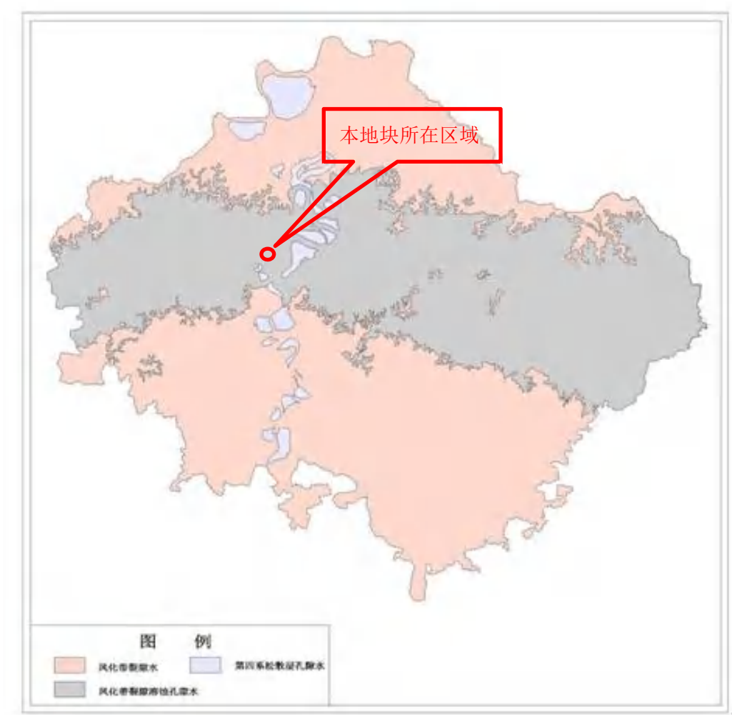
图 3.3-2 雁江区地下水类型分区图
