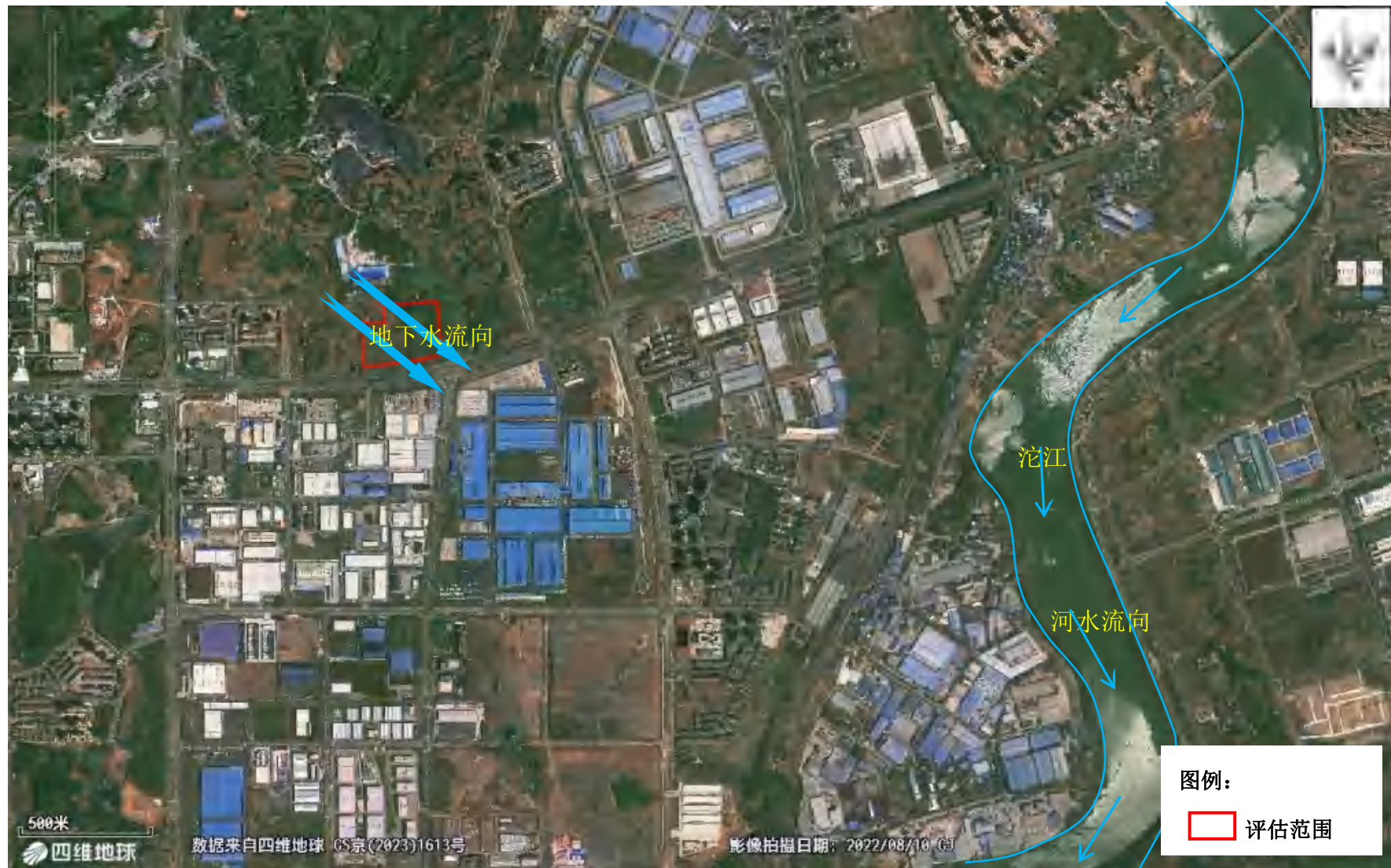
图 4.2-1 评价区域地下水流向
