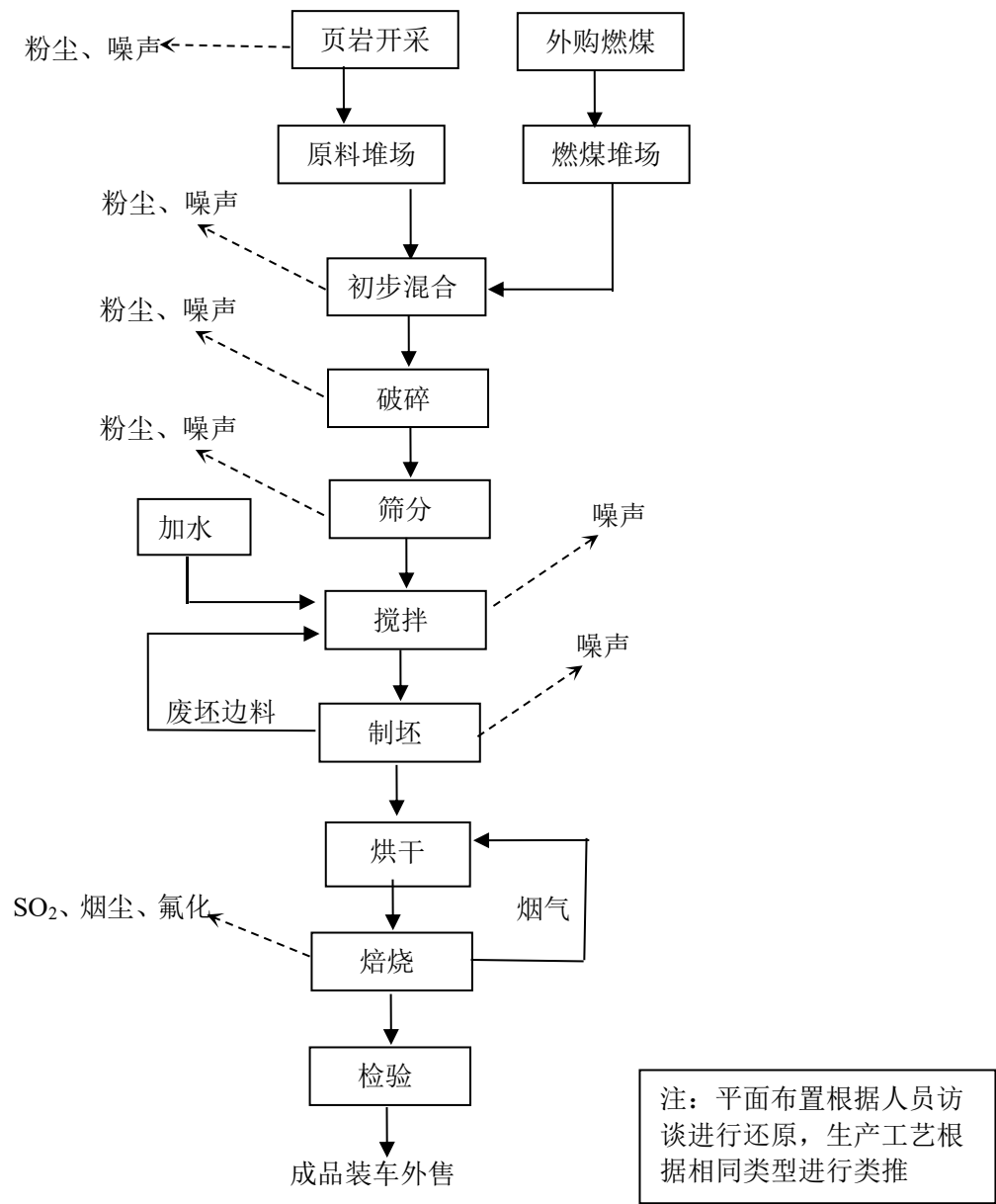
图 6.1-1 生产流程图
