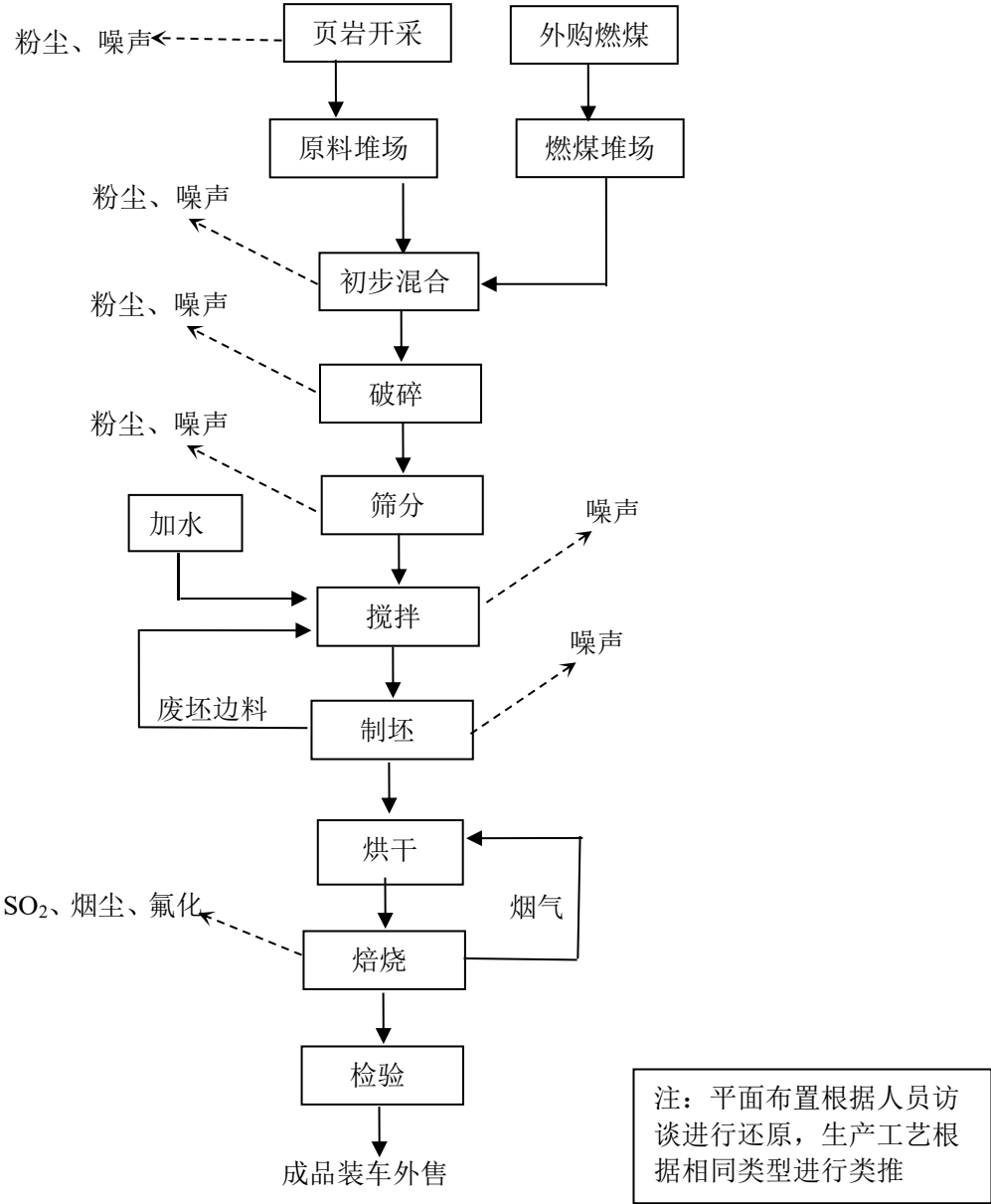
图 6.1-1 生产流程图
