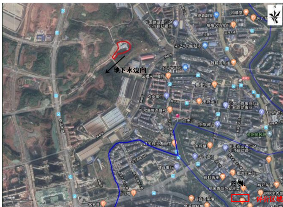
图3.2-1 本项目地下水流向
