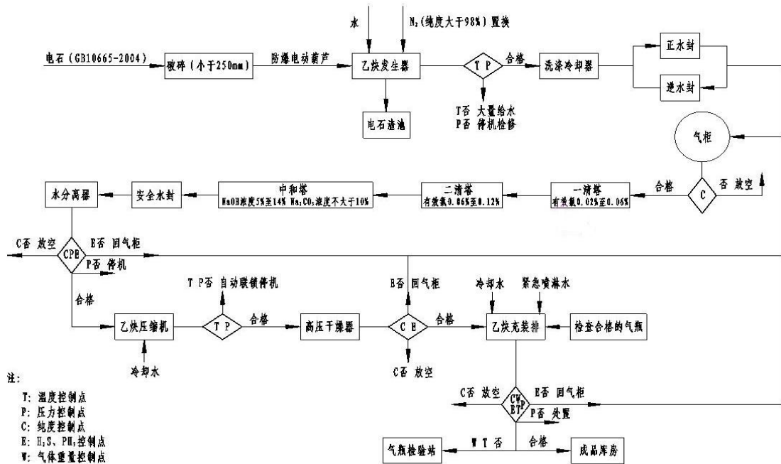
图4.1-1 项目生产工艺流程图
