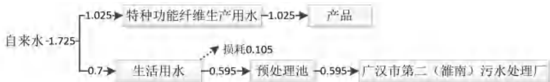
图 2-1 项目水量平衡图(单位: m³/d)
