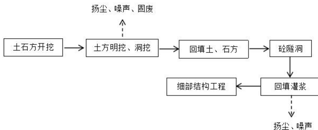
图 4-2 隧洞和暗涵施工工艺流程及产污位置图
