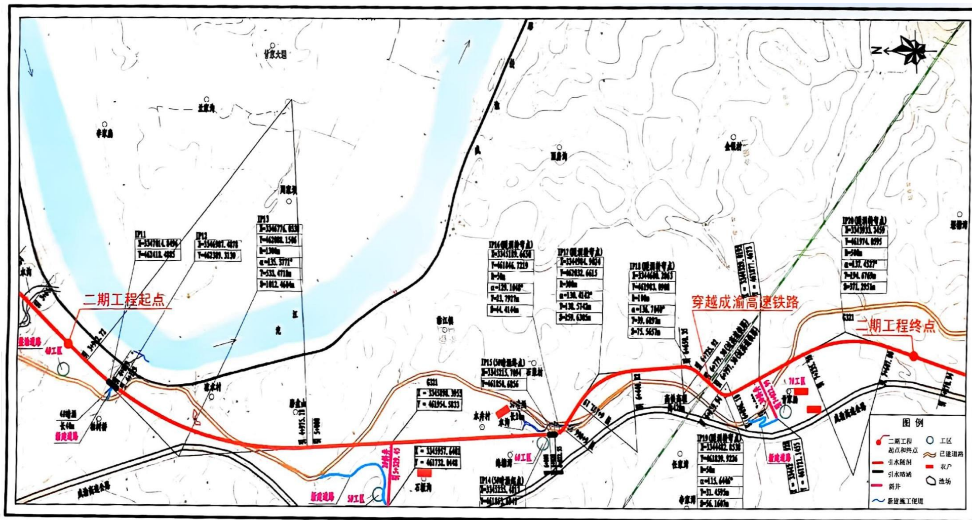
附图二 平面布局及外环境关系图
