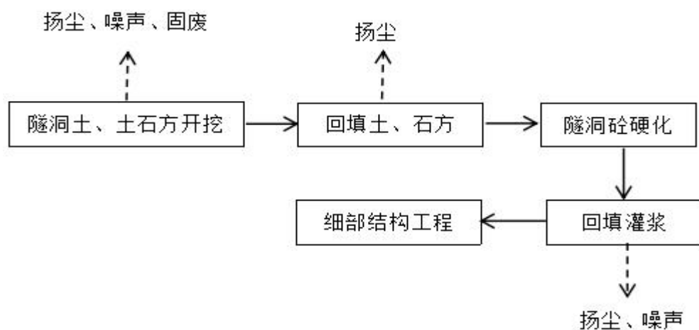
图 4-1 隧洞施工工艺流程及产污位置图
