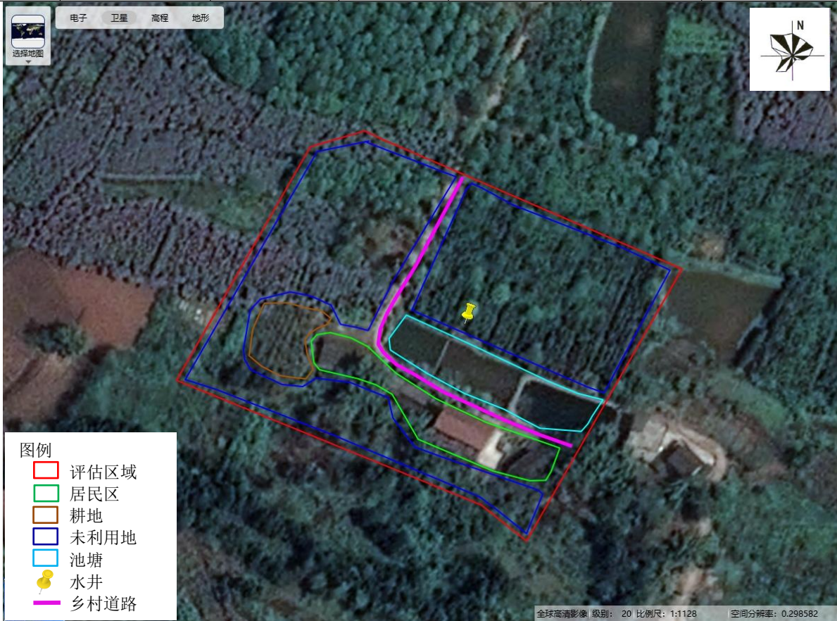
图 3.5-1 地块内平面布局图
