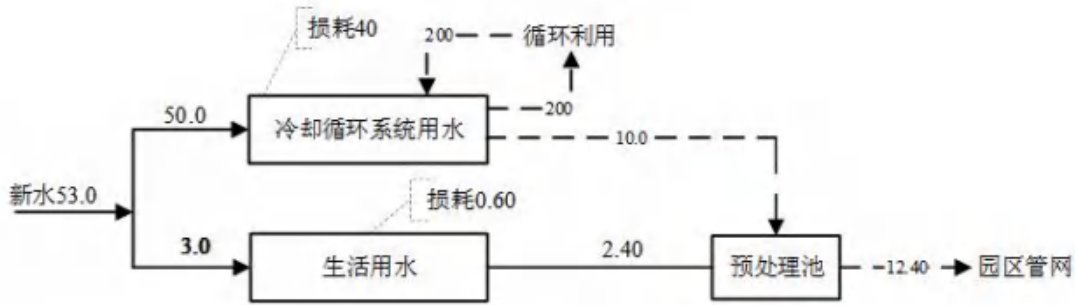
图 3-1 项目水平衡图 (m³/d)
