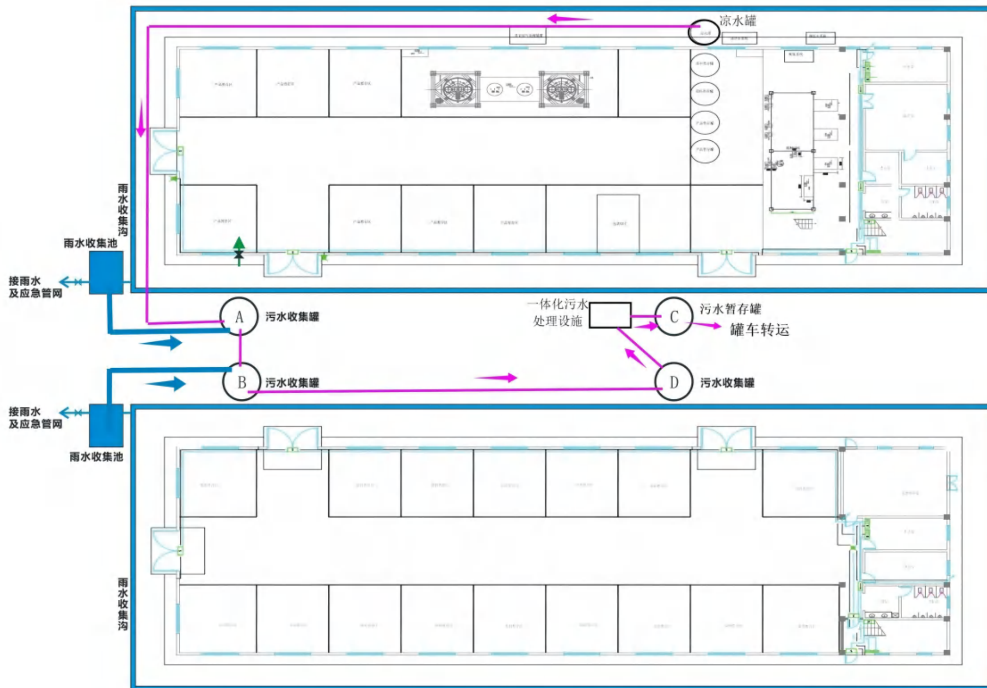
附图4 厂区雨污管线图
