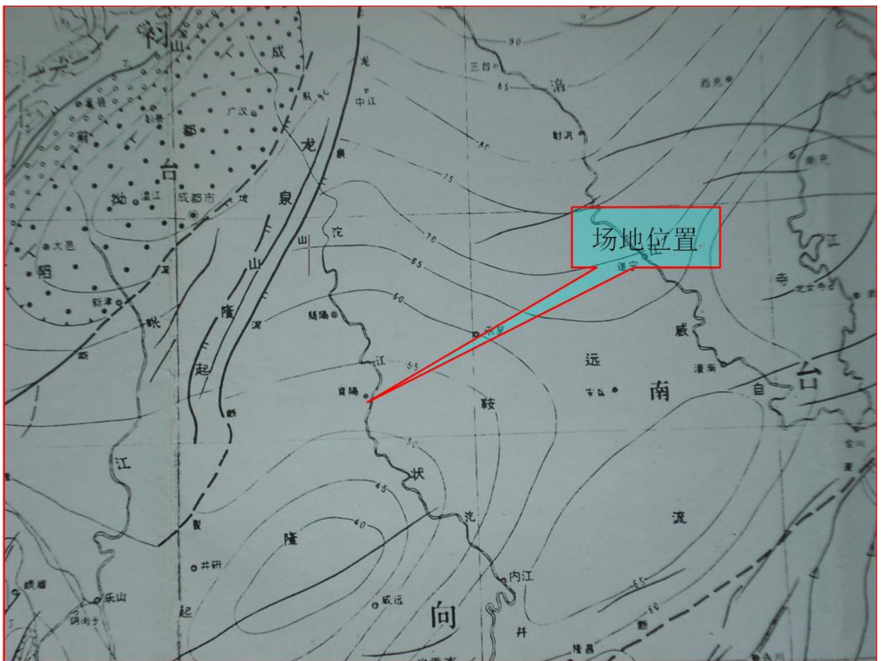
图 3.3-2 区域构造图
